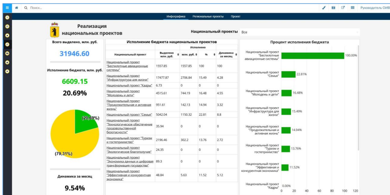
Рисунок 6 – Вкладка «Инфографика»
