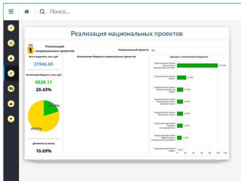
Рисунок 4 – Макеты дашбордов
