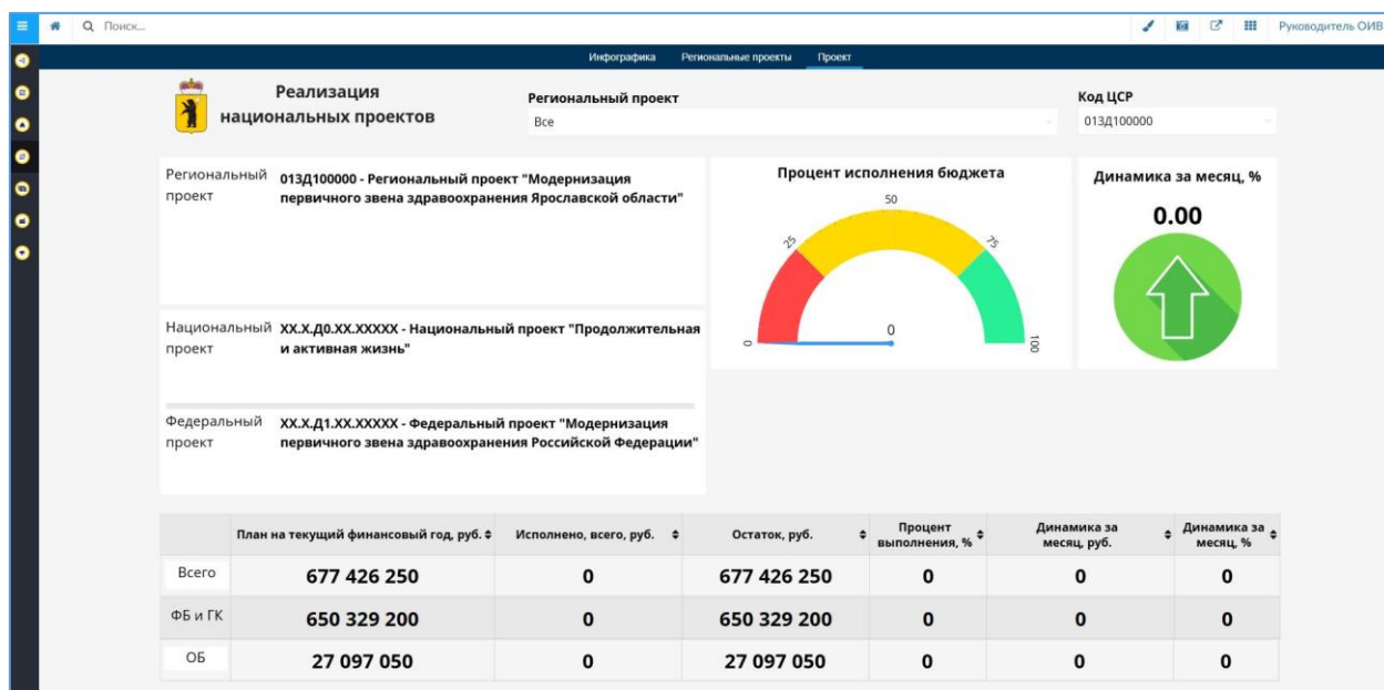
Рисунок 10 – Вкладка «Проект»
